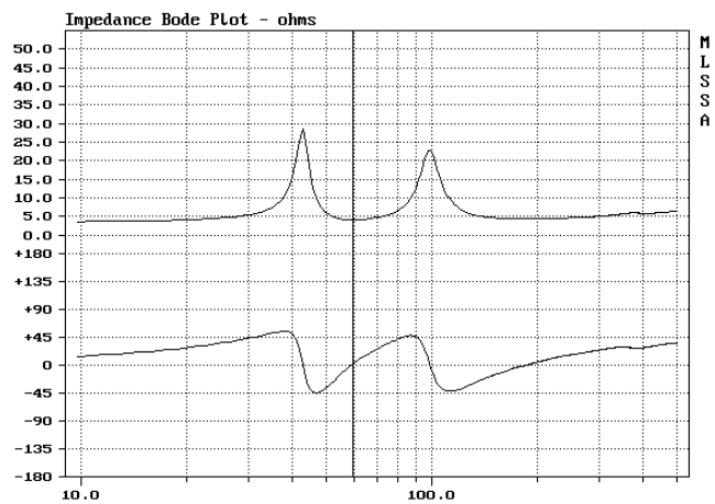
Impedanzverlauf (152Atue)
