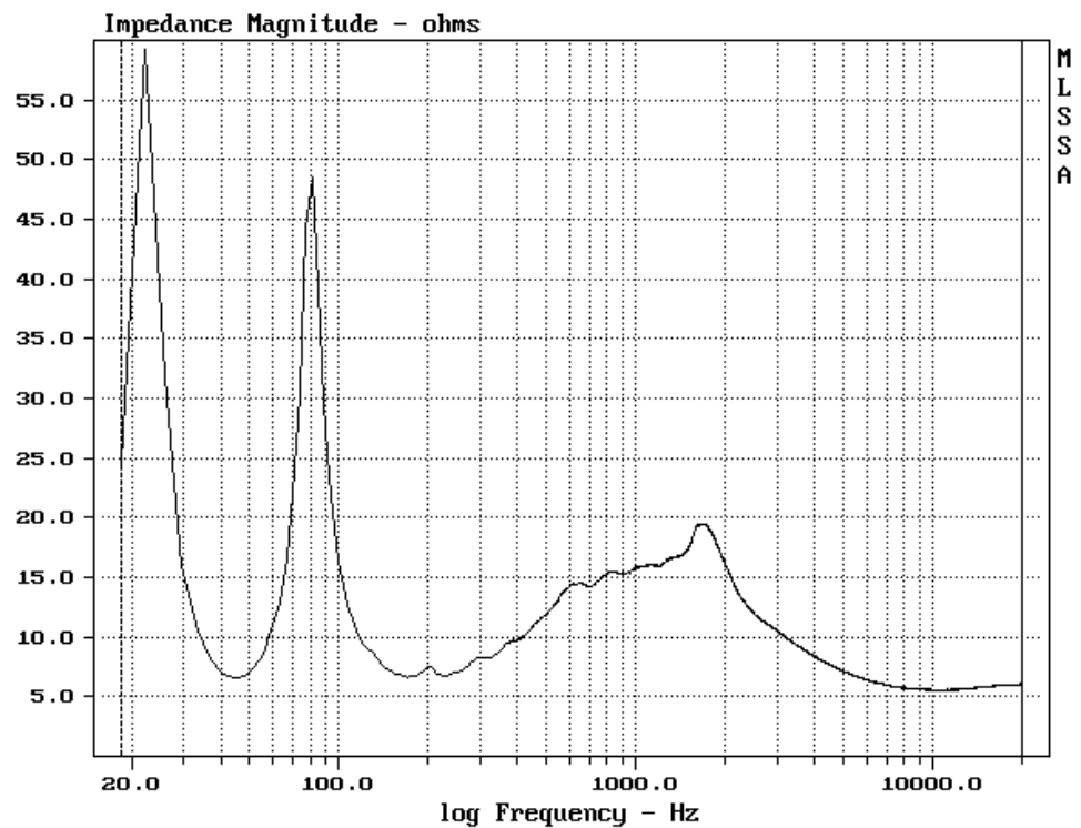
GAE ProStage PS151M Impedanzverlauf / Impedance Plot
